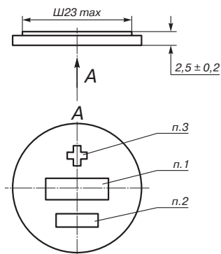
Рис. 1.6. Габариты и маркировка литиевых элементов
