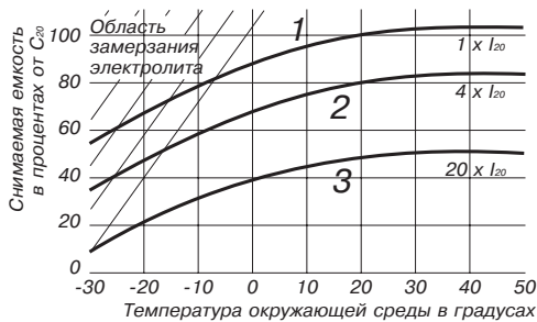
Рис. 2.18. Остаточная снимаемая емкость при разряде постоянным током
